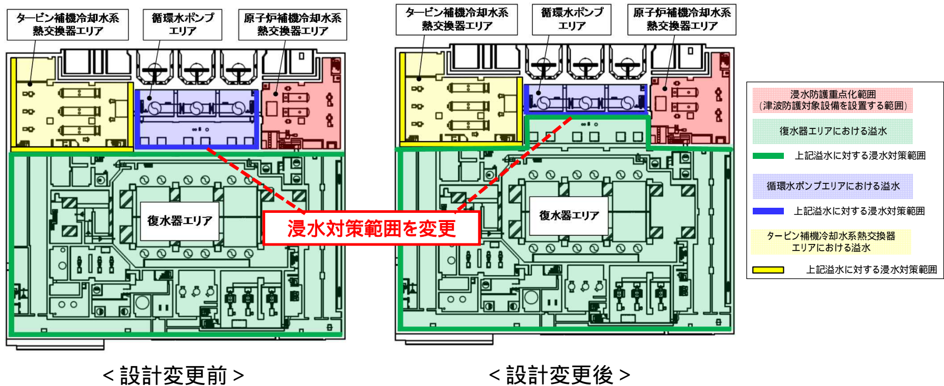
設計変更前後の循環水ポンプエリアと復水器エリアの境界壁 (6号炉タービン建屋地下2階の例)
