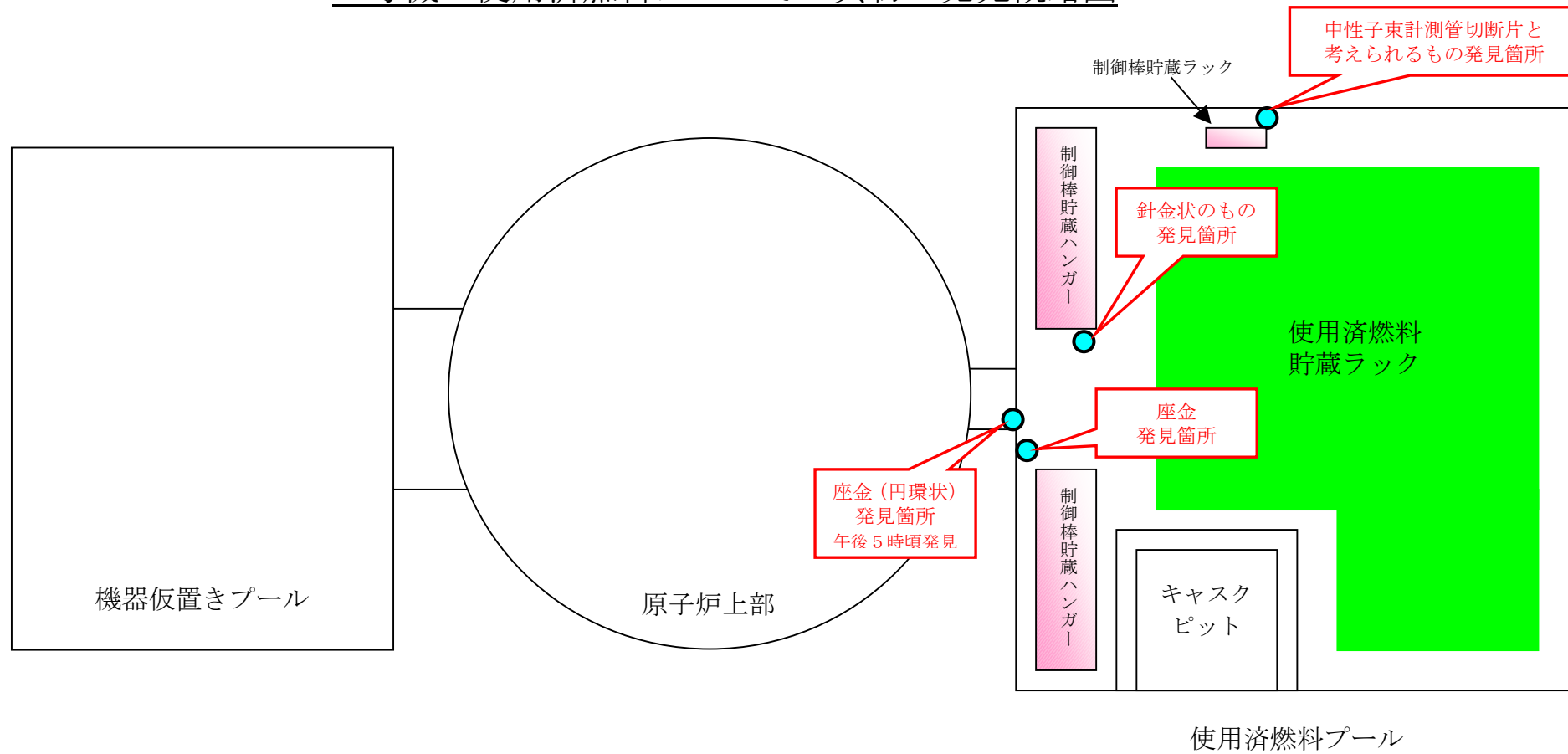
原子炉建屋3階平面図
