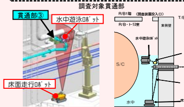
トラス室東側断面調査イメージ
