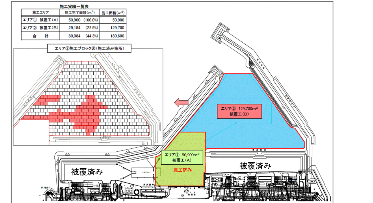
図9：港湾内海底土被覆の進捗状況
