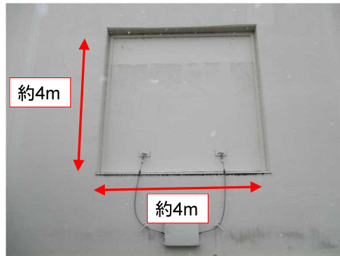
ブローアウトパネル外観
