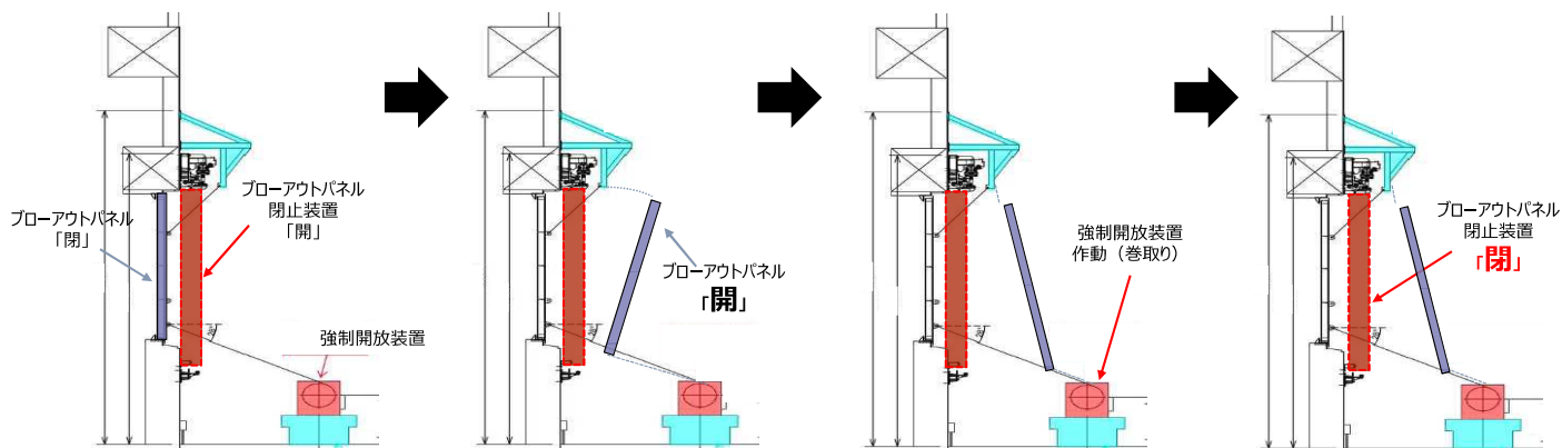
①ブローアウトパネル通常時
