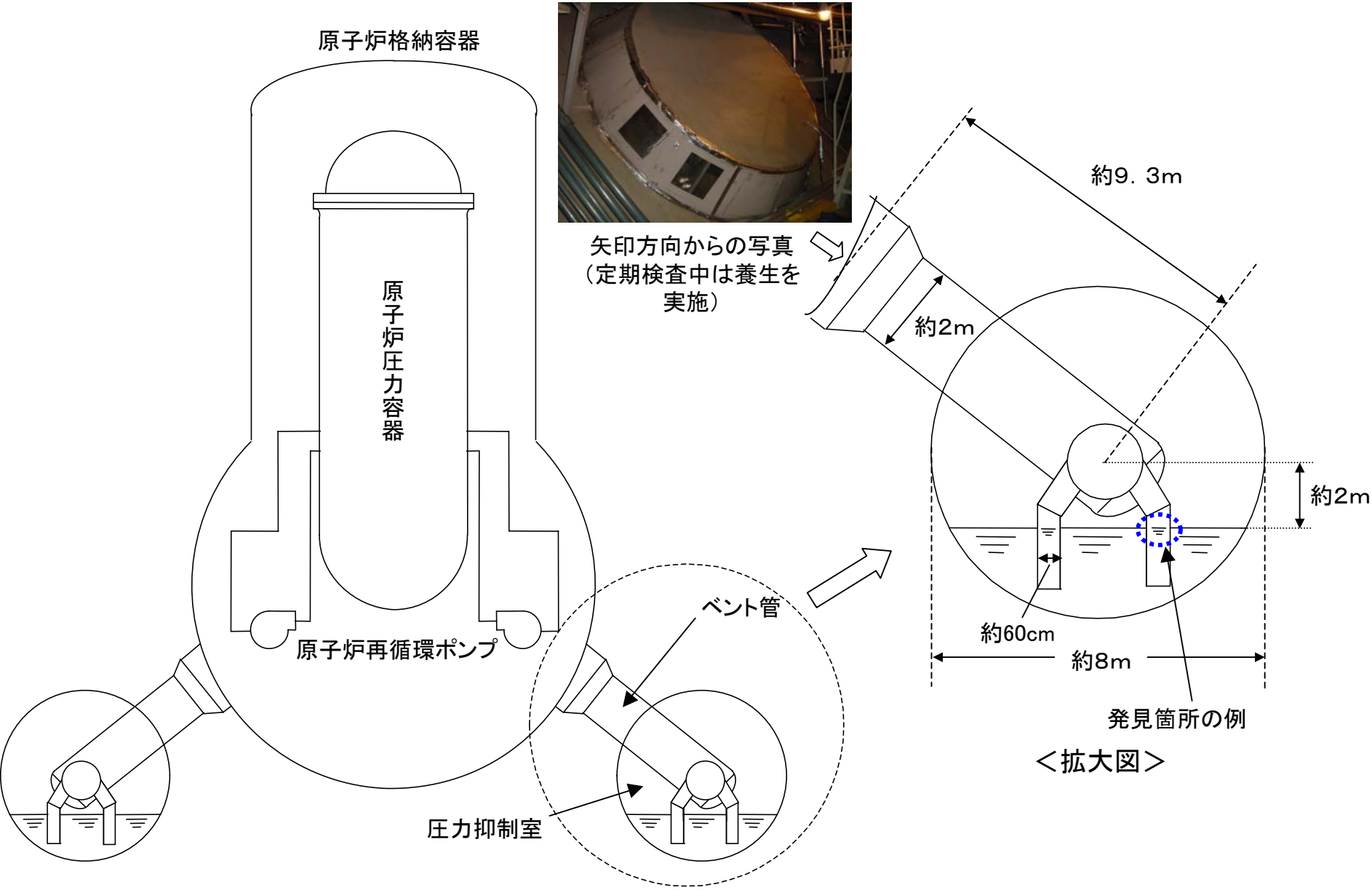
4号機圧力抑制室ベント管内でのシート片発見概要図
