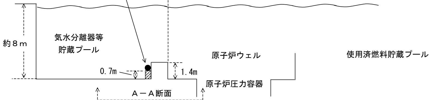
原子炉建屋5階断面図
