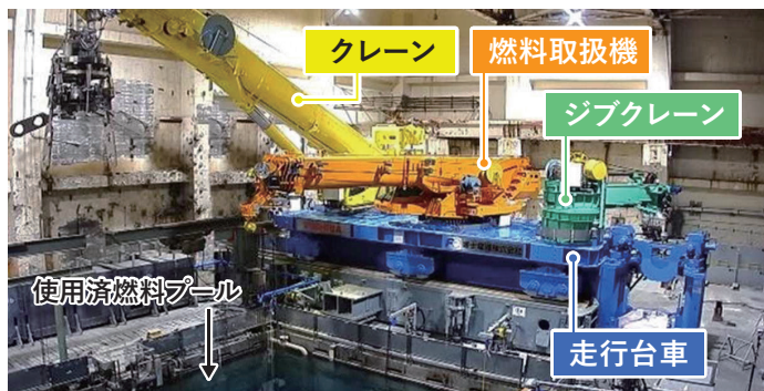
2号機 原子炉建屋内燃料取扱設備全景（遠隔監視カメラにて撮影）
