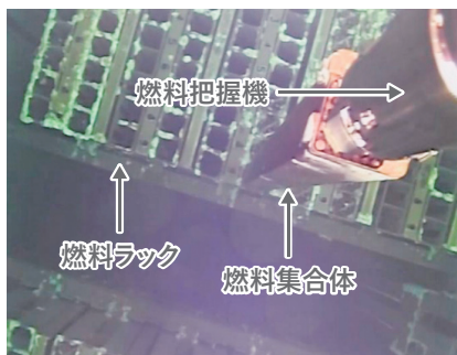
ラックから燃料集合体を引き上げている様子
