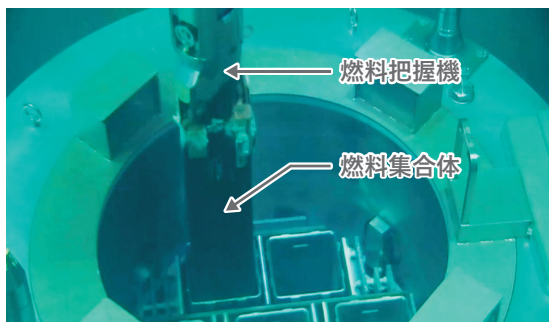
キャスク ※2 へ燃料集合体を収納している様子
