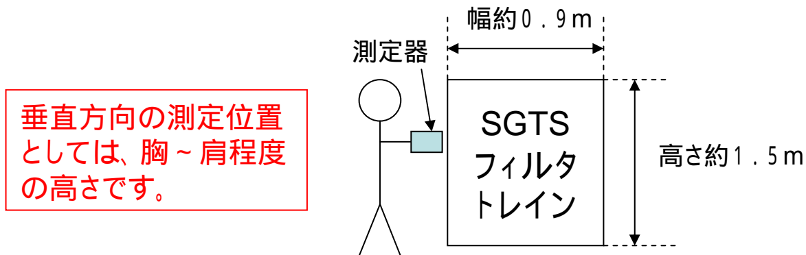
SGTSフィルタトレインの線量測定方法
