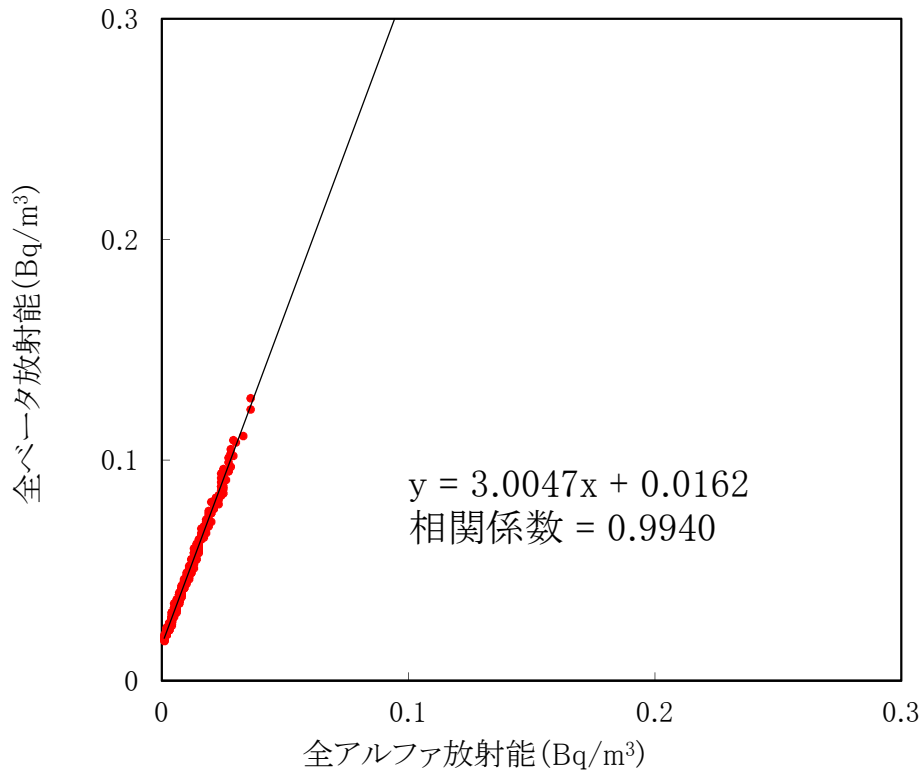
大気浮遊じんの全アルファ・全ベータ放射能の相関図 (MP-1) (令和4年10月～令和4年12月)
