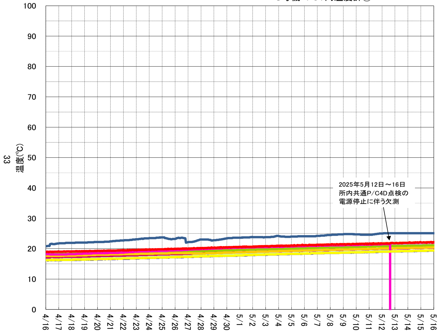
3号機 PCV内温度計②
