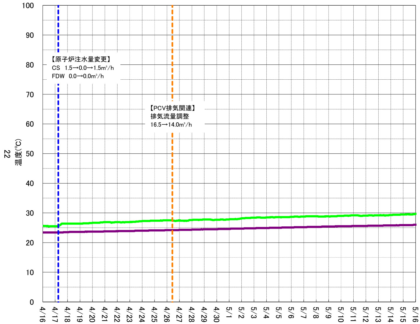
2号機 実施計画関連温度計(RPV)
