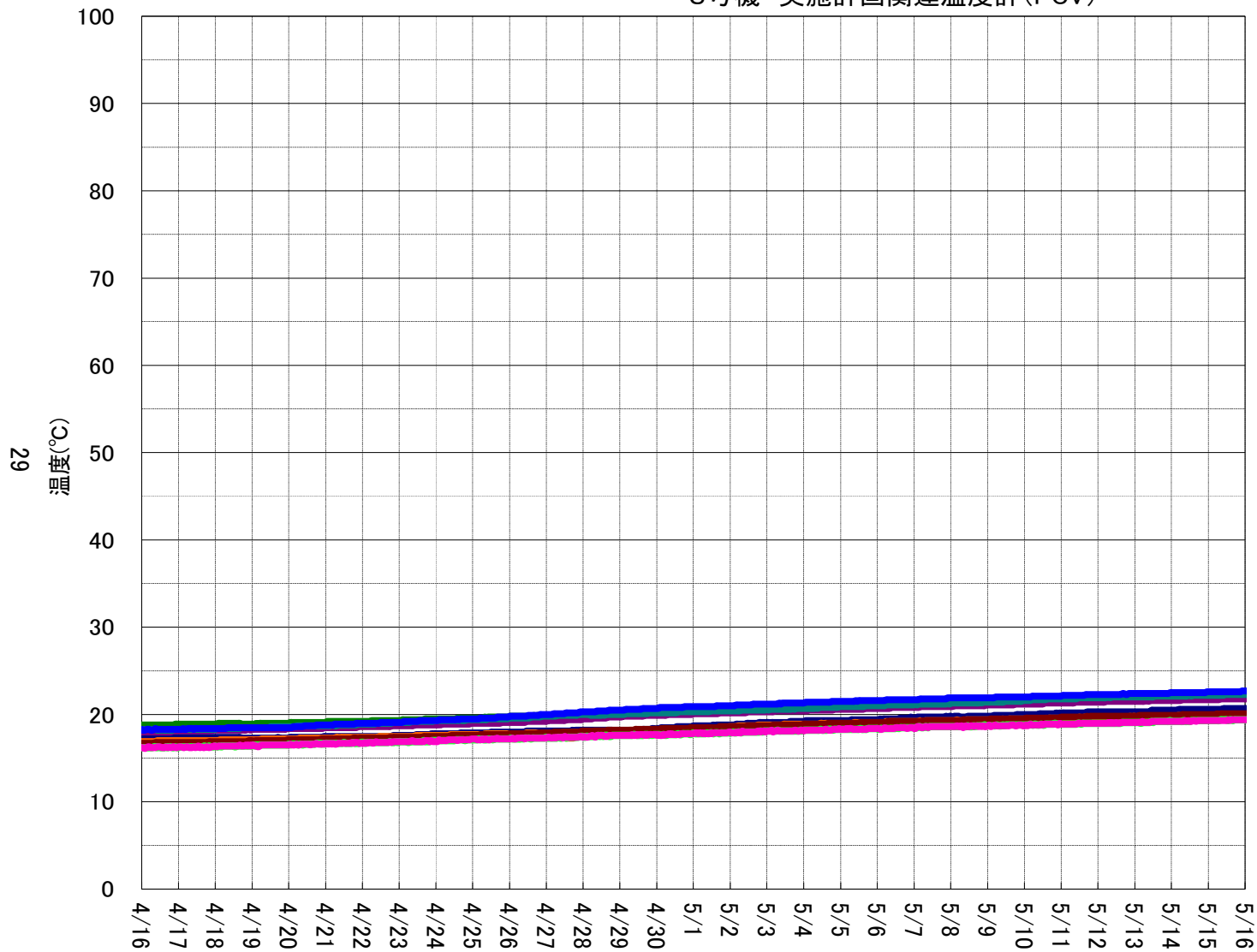
3号機 実施計画関連温度計(PCV)
