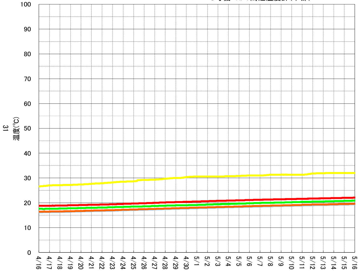
3号機 RPV周辺温度計(下部)
