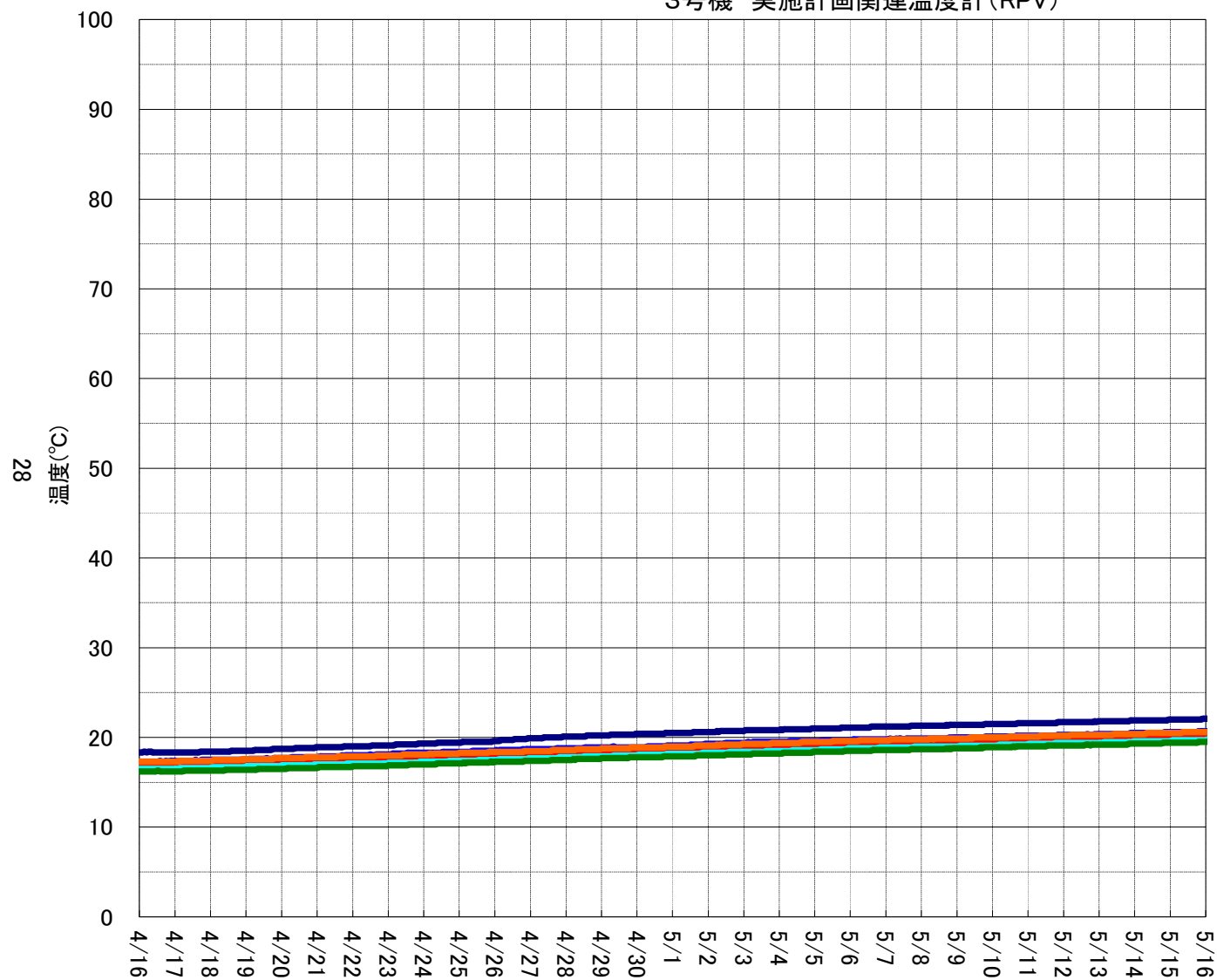
3号機 実施計画関連温度計(RPV)
