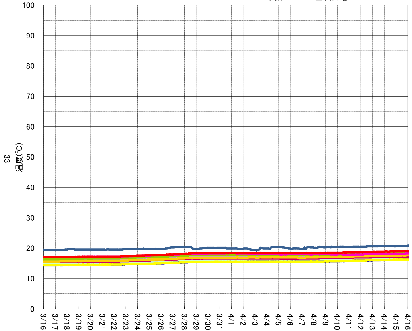
3号機 PCV内温度計②
