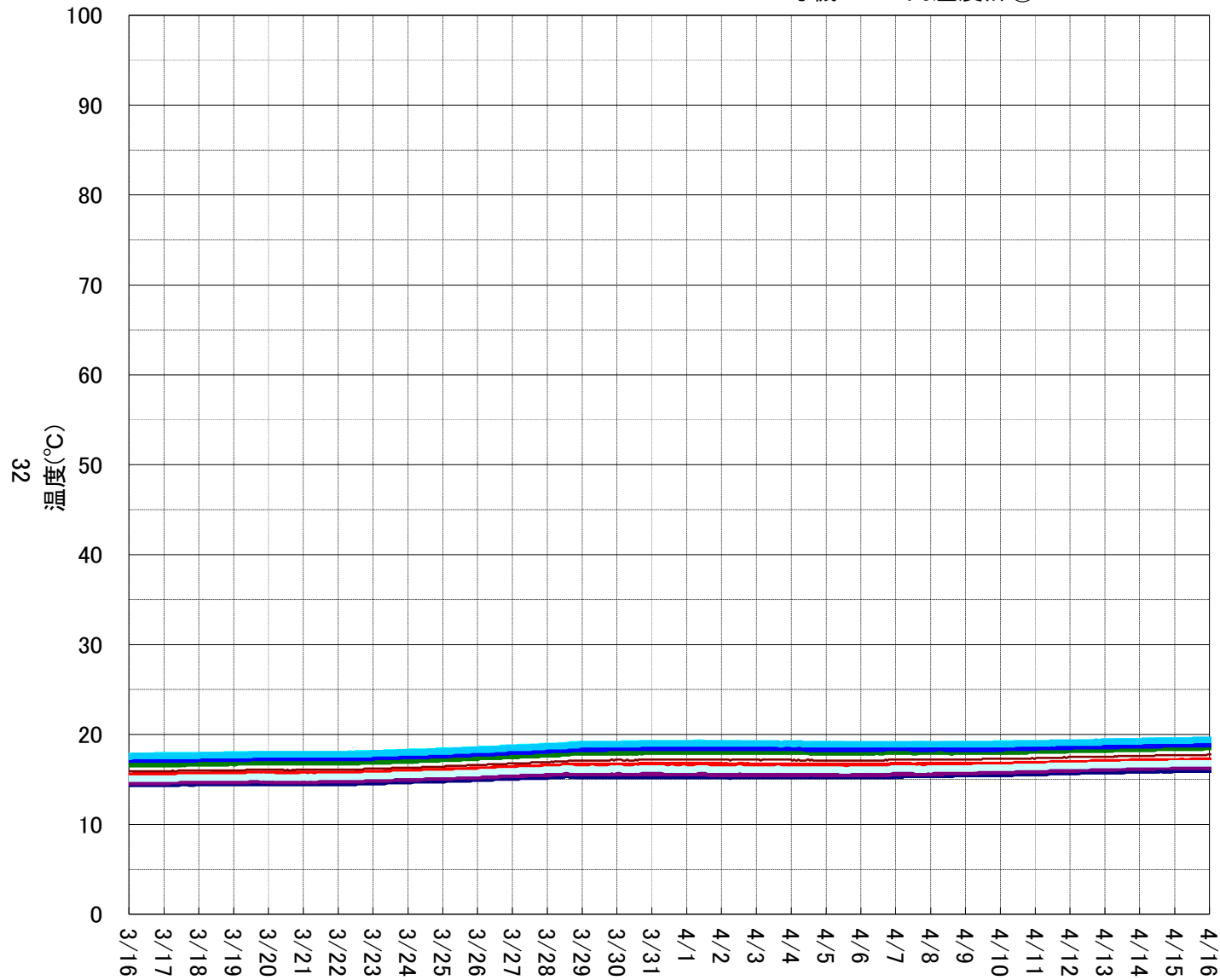
3号機 PCV内温度計①
