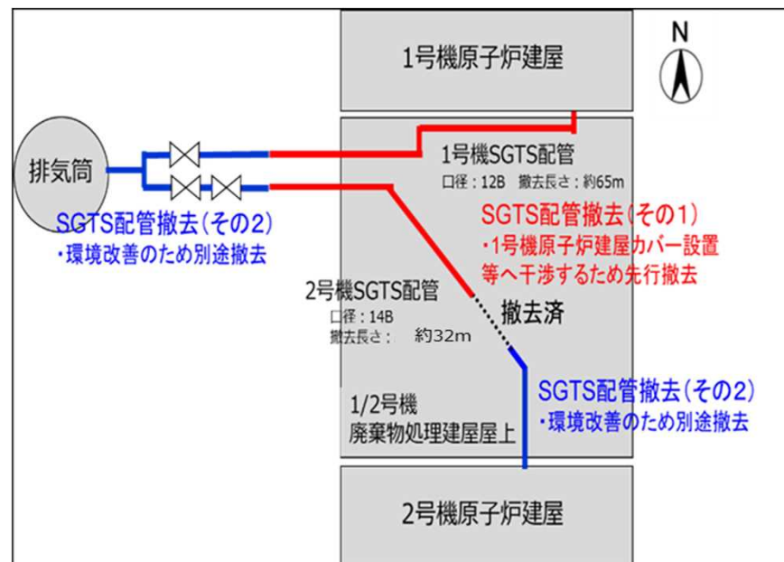
SGTS配管撤去（その1）の作業範囲
