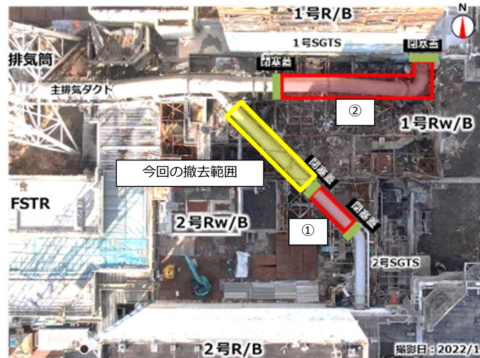
1・2号機廃棄物処理建屋主排気ダクト
