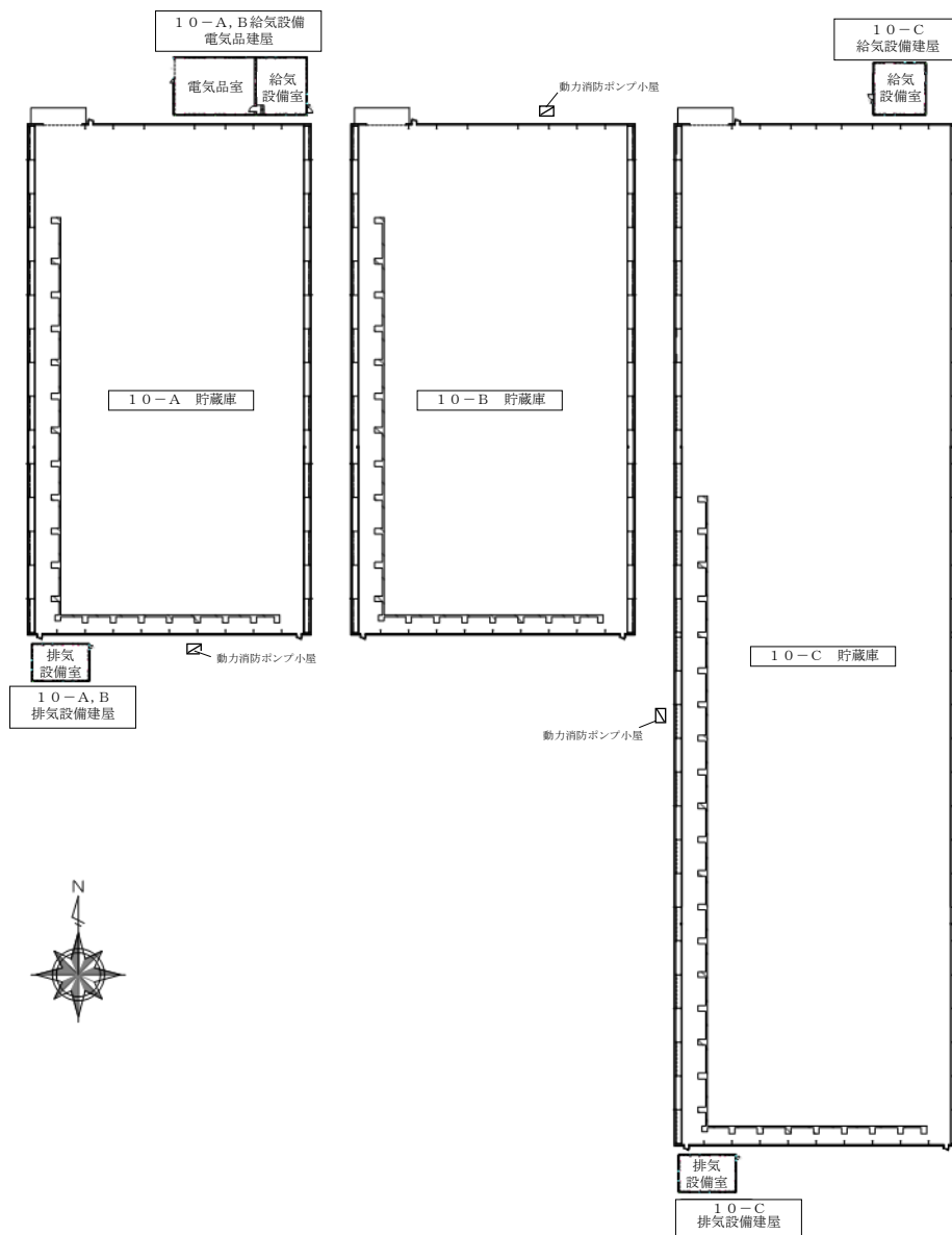
図-4 固体廃棄物貯蔵庫第10棟の平面図
