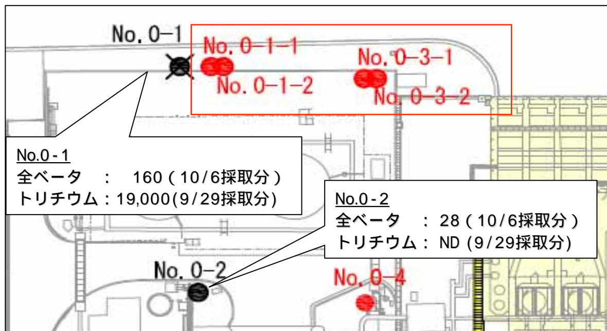
施工位置図
