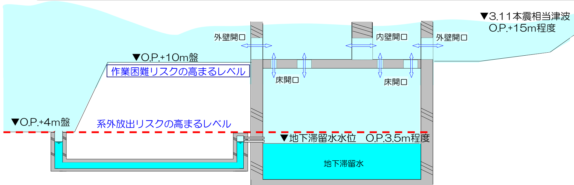
建屋への津波流入経路概略図
