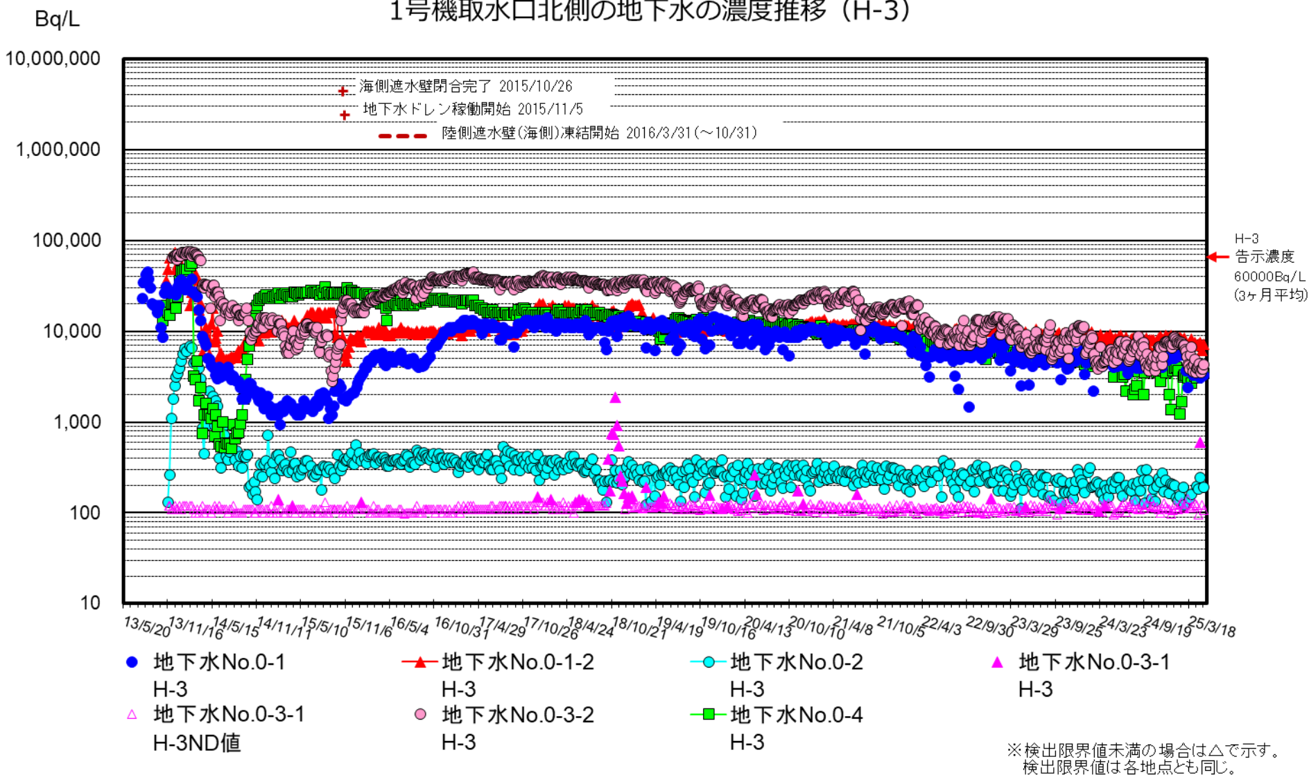
1号機取水口北側の地下水の濃度推移 (H-3)
