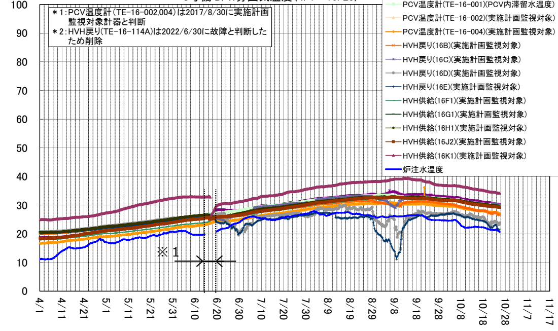
3号機 D/W雰囲気温度 (4/1~10/25)
