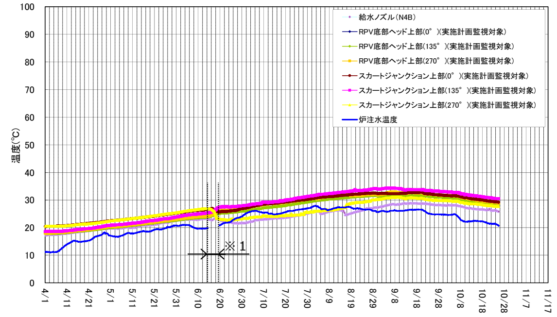
3号機 原子炉压力容器まわり温度 (4/1~10/25)
