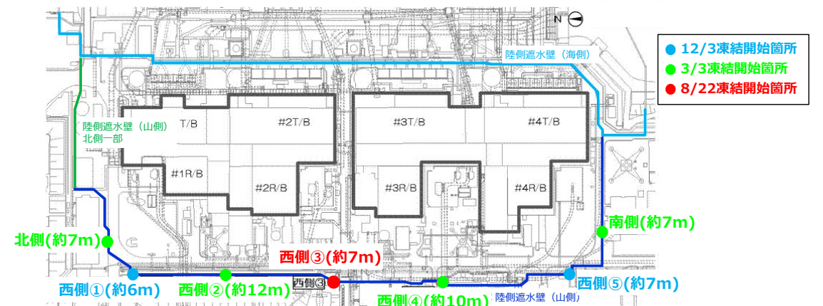
図2：陸側遮水壁（山側）の閉合箇所
