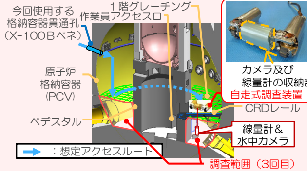
格納容器内調査イメージ
