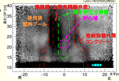
ミュオン測定により<原子炉建屋を透視した様子>
