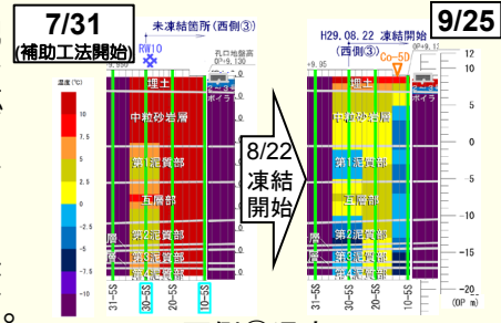
<西側③温度>
