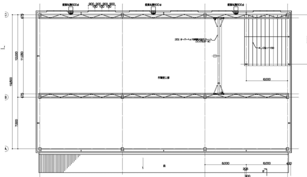
1階上部平面図
