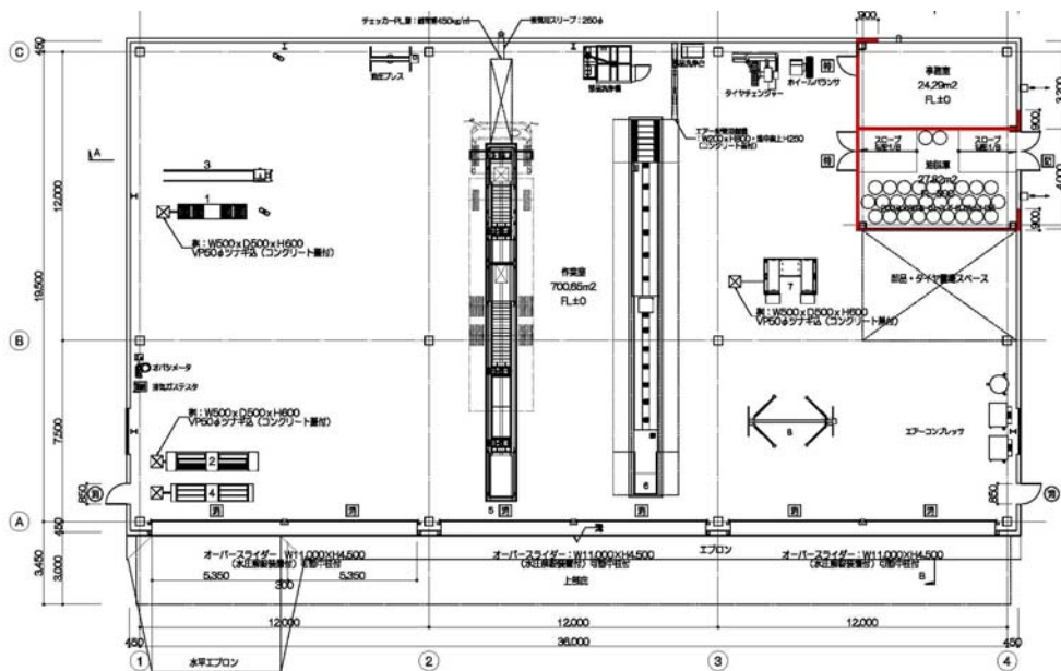
1階平面図
