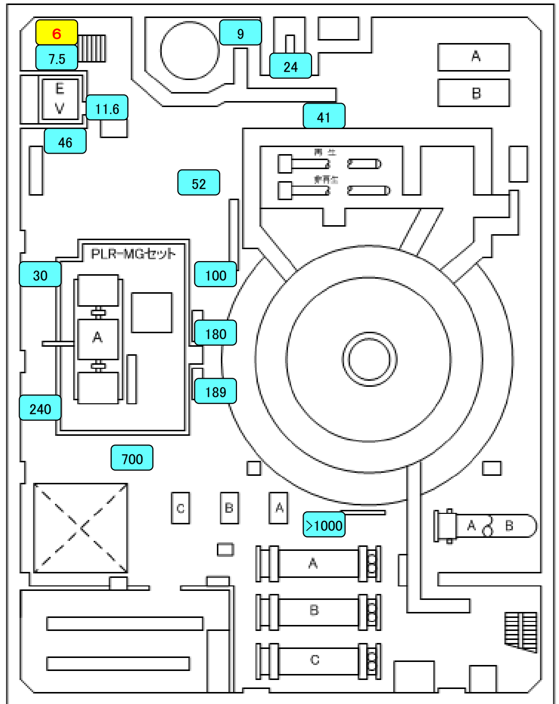
1号機 原子炉建屋 2階
