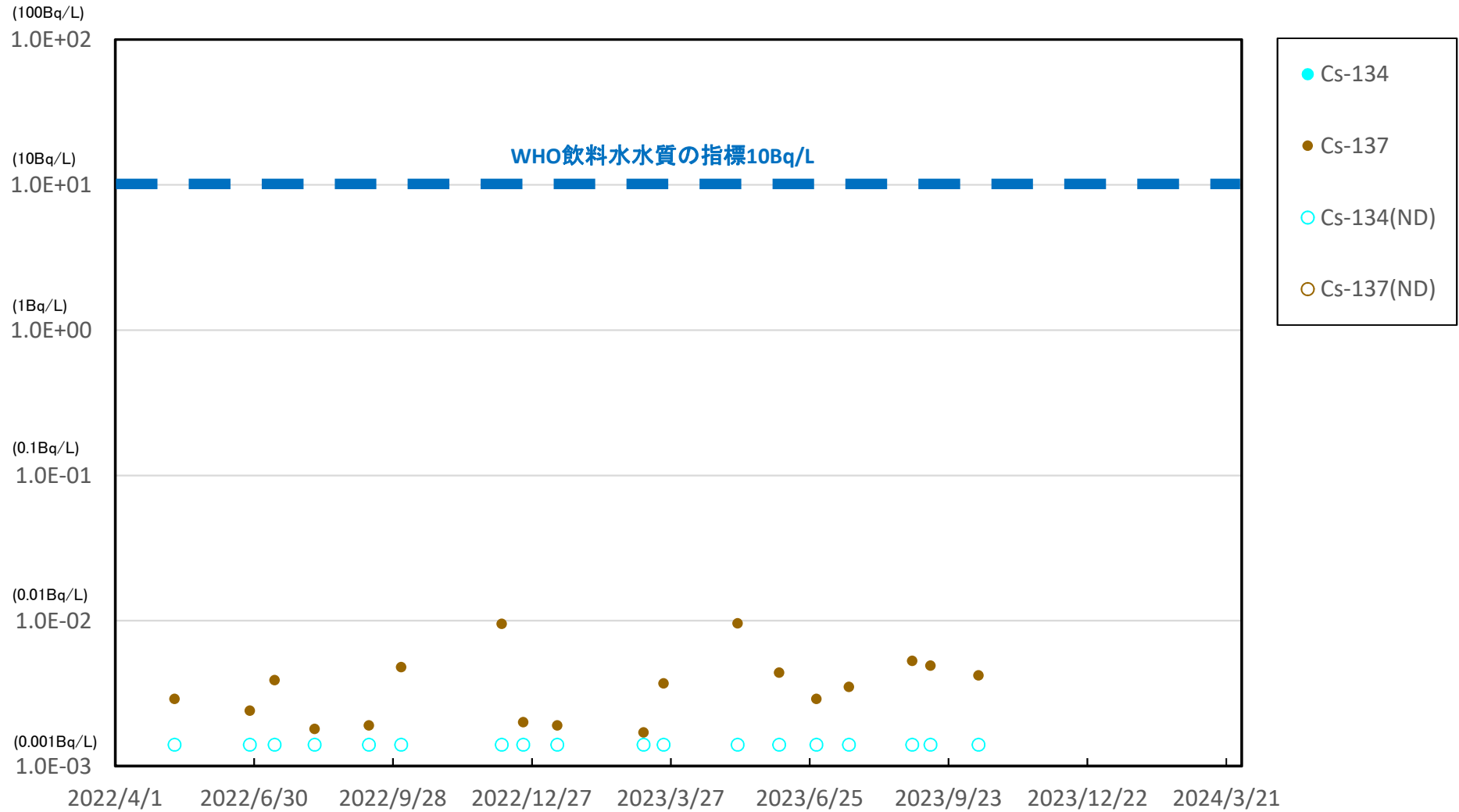
熊川沖合4km付近(T-S8) 底層 海水放射能濃度
