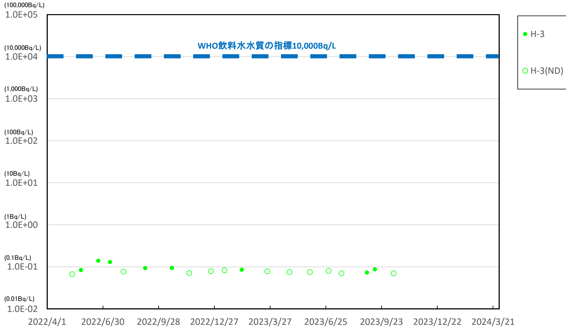
福島第一 敷地沖合3km付近(T-S4) 表層 海水放射能濃度
