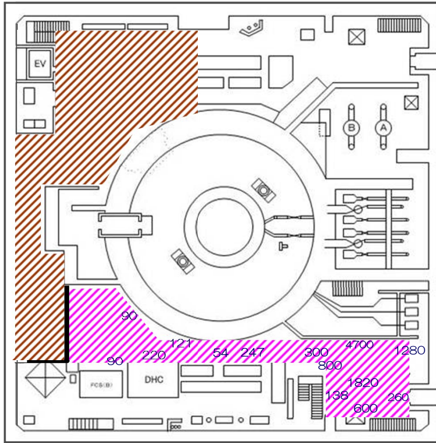
1号機1階
