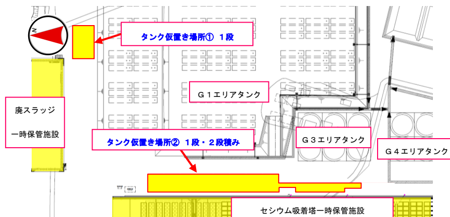
図－2 濃縮水受タンク・濃縮処理水タンクの仮置き場所
