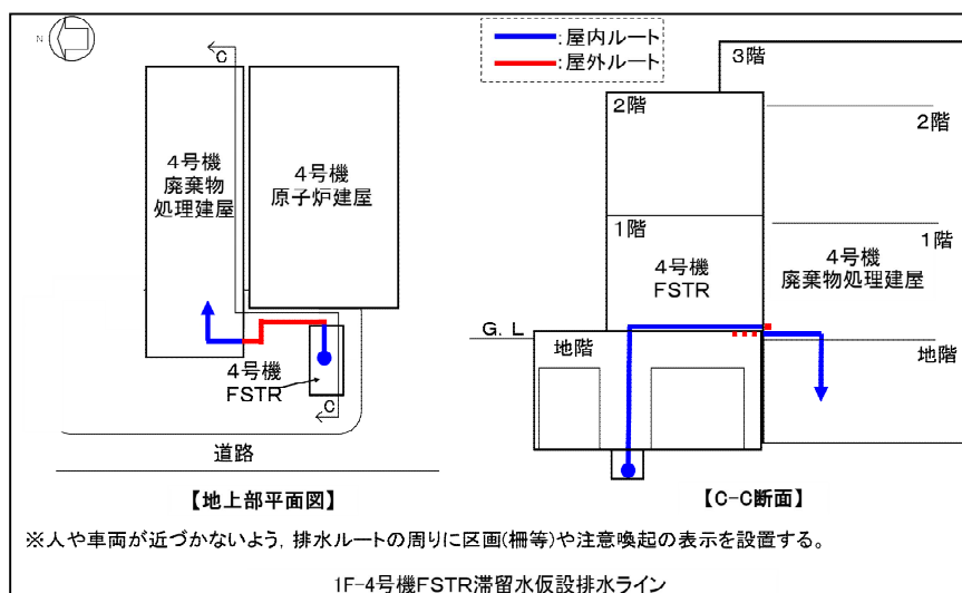
図ー 2 屋外排水ライン図
