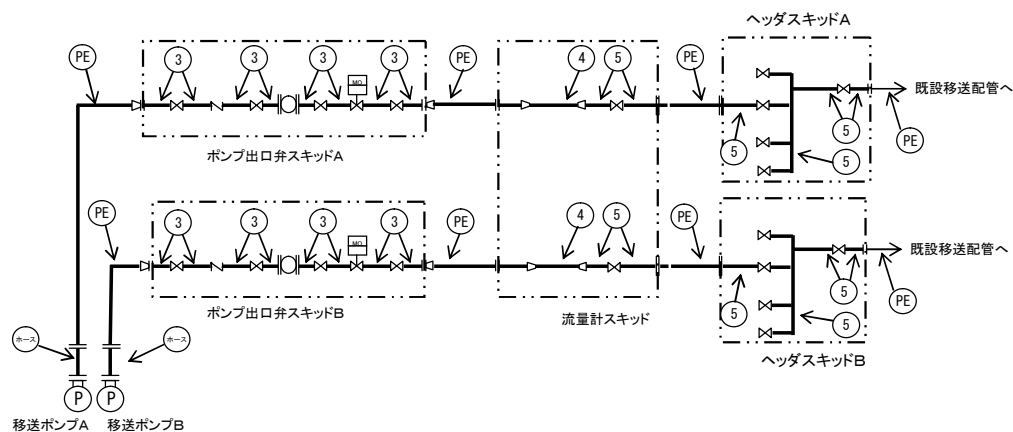
図－1 配管概略図（2／2）
