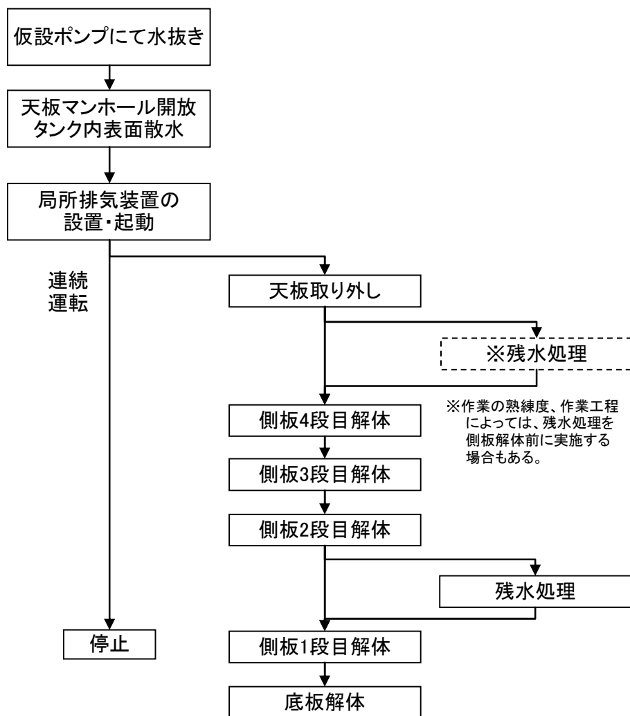
図－１３ 解体作業のフロー
