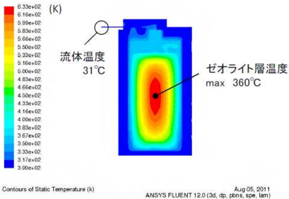
図ー 1 3次元解析計算によるセシウム吸着装置吸着塔の温度分布
