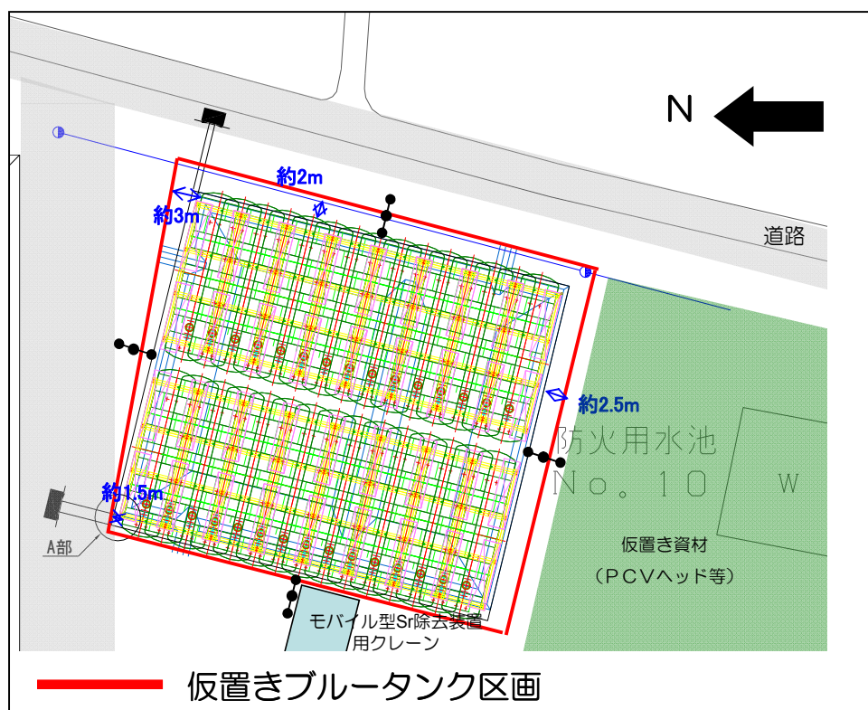
図－４ ブルータンクエリアA区画图
