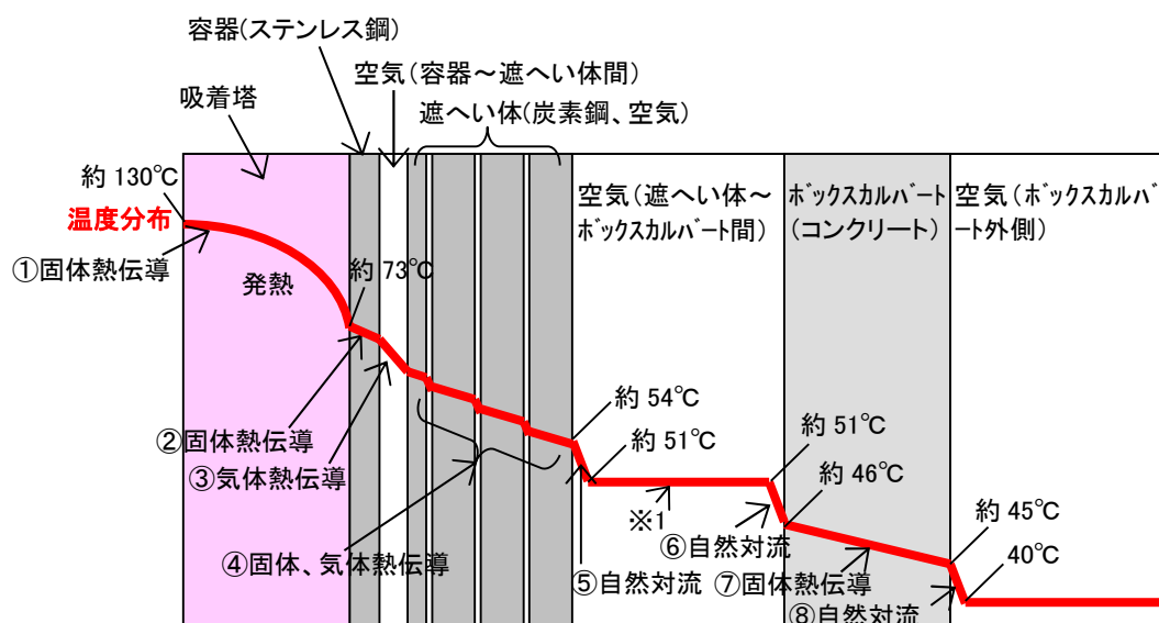
図－１ 評価体系の概念図（１次元定常温度評価モデル）および温度分布（吸着塔）
