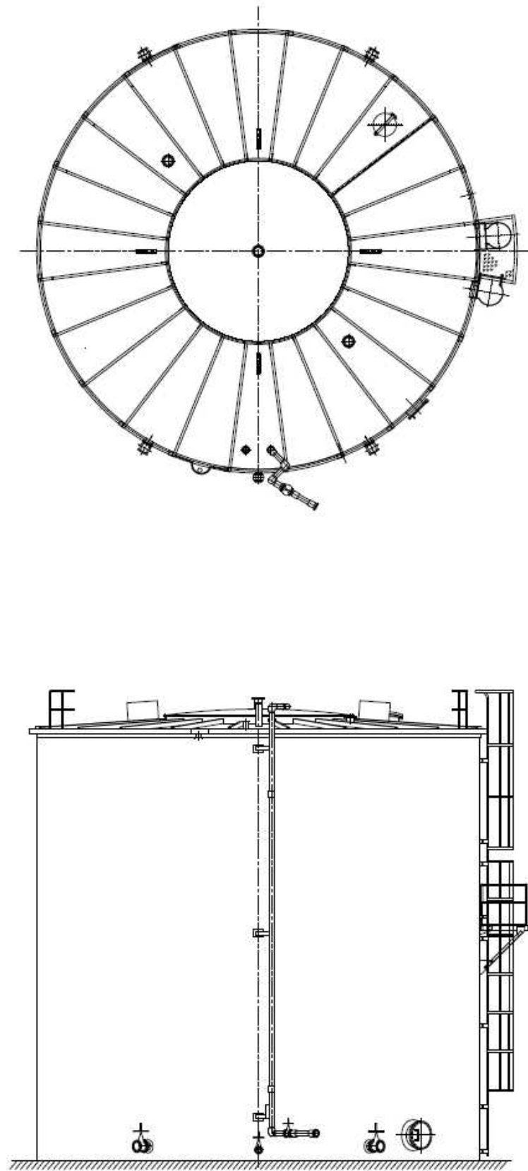
溶接型タンク概略図 (H1)
