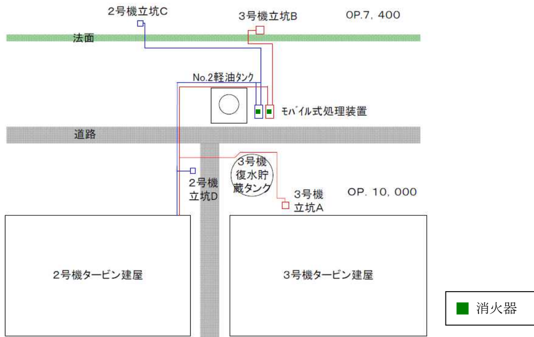
図 2 配置概要図
