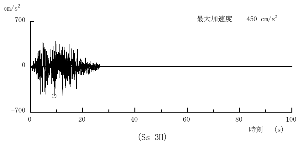
図一 8 解放基盤表面位置における地震動の加速度時刻歴波形（水平方向）
