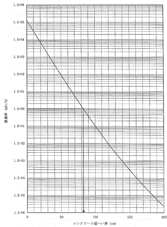
図ー 4 スラッジ貯槽周りのコンクリート遮へい厚と壁外表面の線量率の関係（軸方向）
