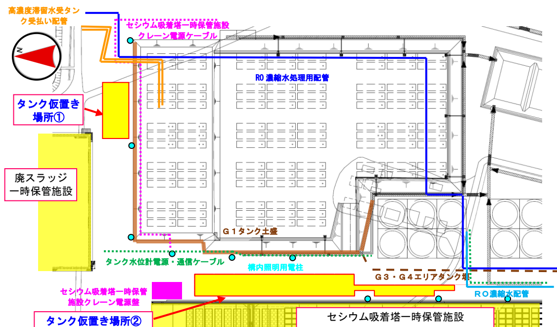
図ー４ タンク仮置き場所周辺図
