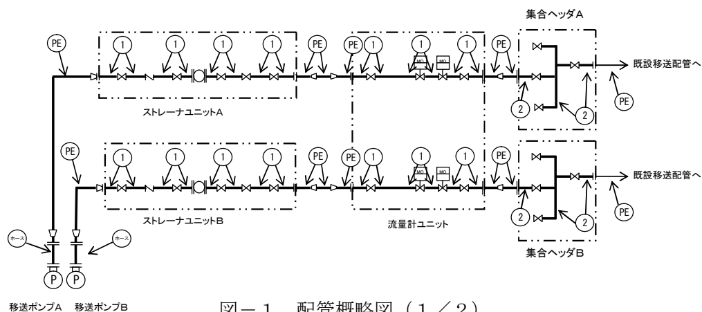
図－１ 配管概略図（１／２）
