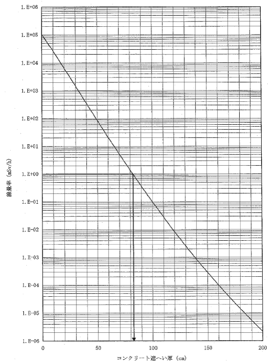
図ー 3 スラッジ貯槽周りのコンクリート遮へい厚と壁外表面の線量率の関係（径方向）
