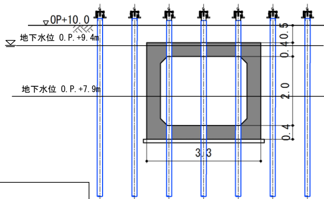
断面図
