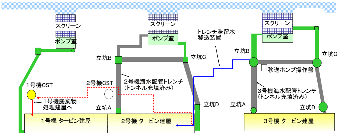
図2 概要図
