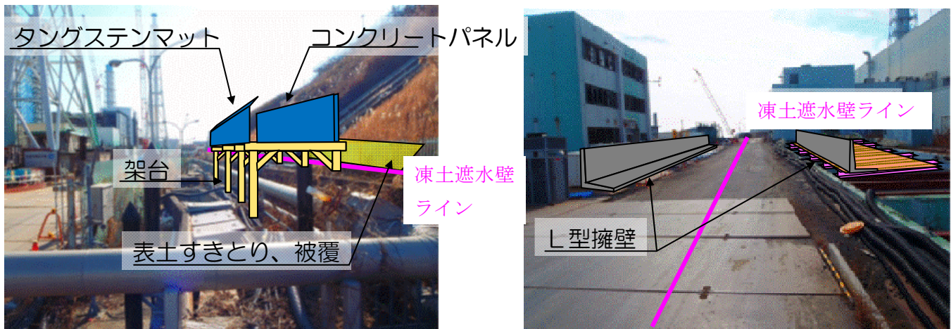
図 1 0 被ばく線量低減対策実施例 1
