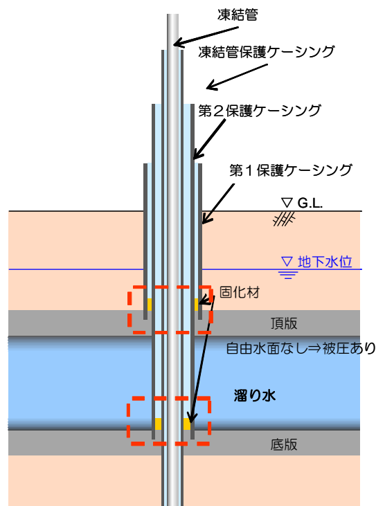
頂版・底版マルチステップ工法 (内部充填工を実施しない場合の例)
