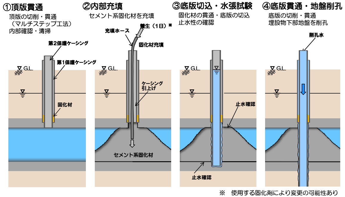
図10 マルチステップ工法の施工手順(頂版マルチステップ・底版内部充填工法のケース)
