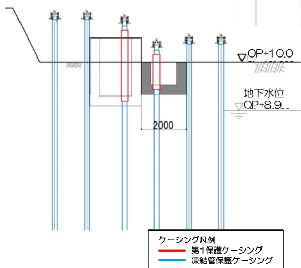
図 1 4 - 5 ケーブルダクト 施工方法 (貫通施工)
