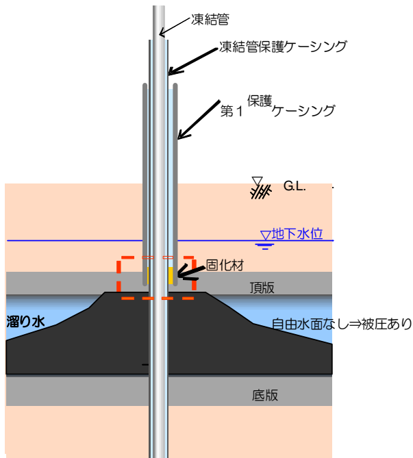
頂版マルチステップ・底版内部充填工法
