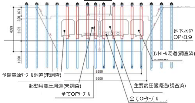
図 1 4 - 7 1号機電気ケーブルダクト 施工方法 (貫通施工)
