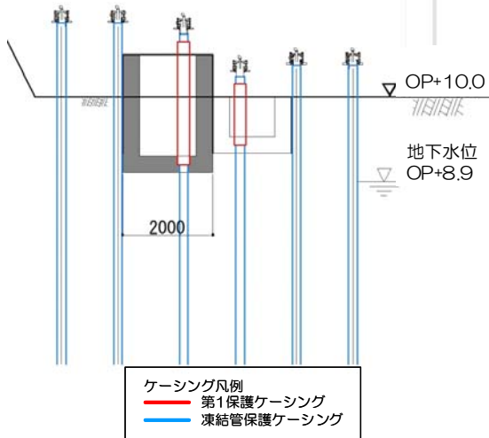
図 1 4 - 6 発電所西側ケーブルダクト 施工方法 (貫通施工)
