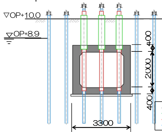
図 1 4 - 1 7 2~4 号機 DG 連絡ダクト① 施工方法 (貫通施工)
