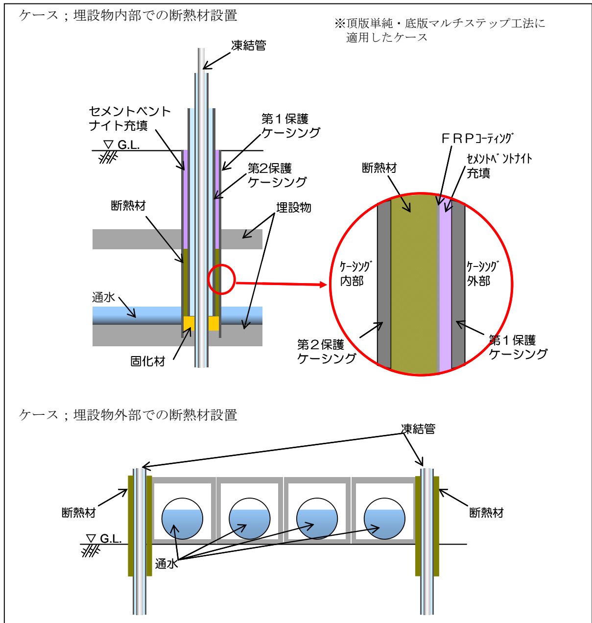
図 1 1 凍結管外周部への断熱材設置による凍結防止
