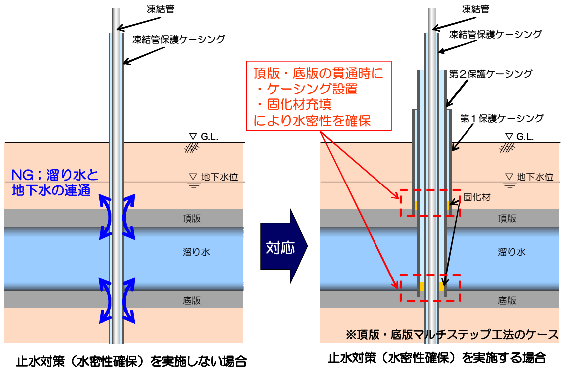
図6 貫通施工時の留意事項
