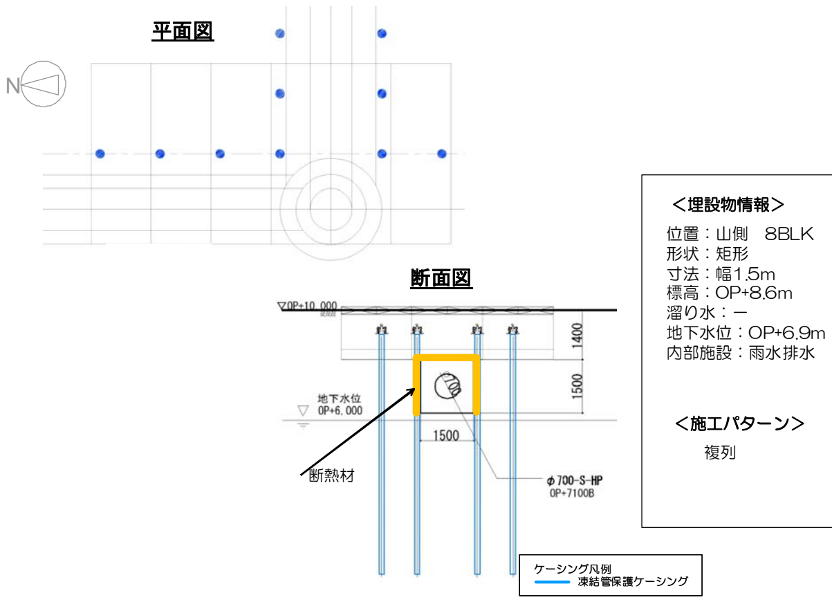
図 1 4 - 2 5 排水ヒューム管③ 施工方法（複列施工）
