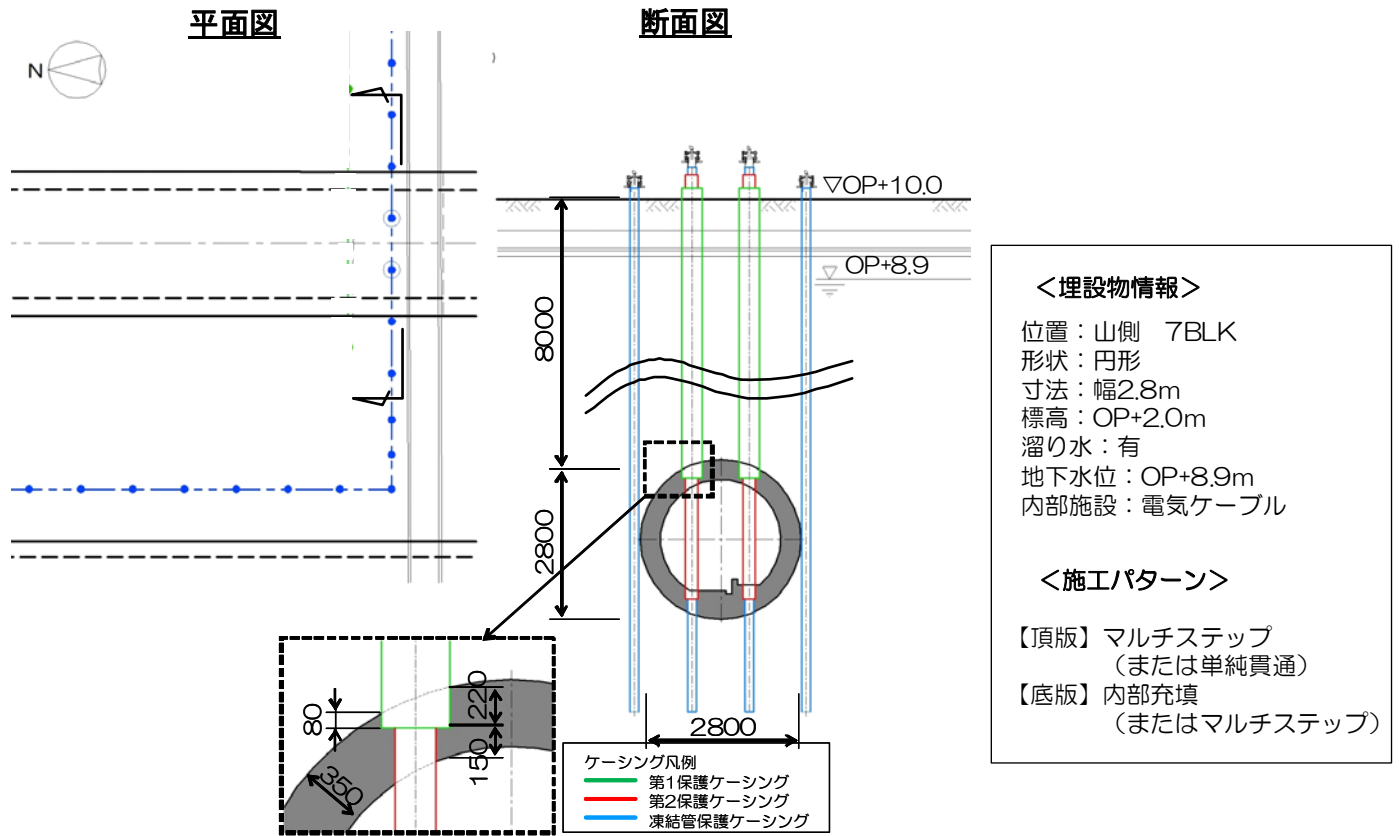
図14-18 2~4号機DG連絡ダクト② 施工方法 (貫通施工)
