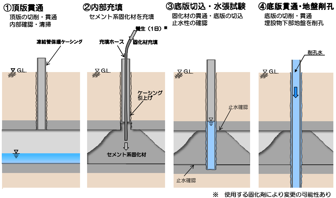
図7 内部充填工法の施工手順（頂版単純貫通・底版内部充填工法のケース）
