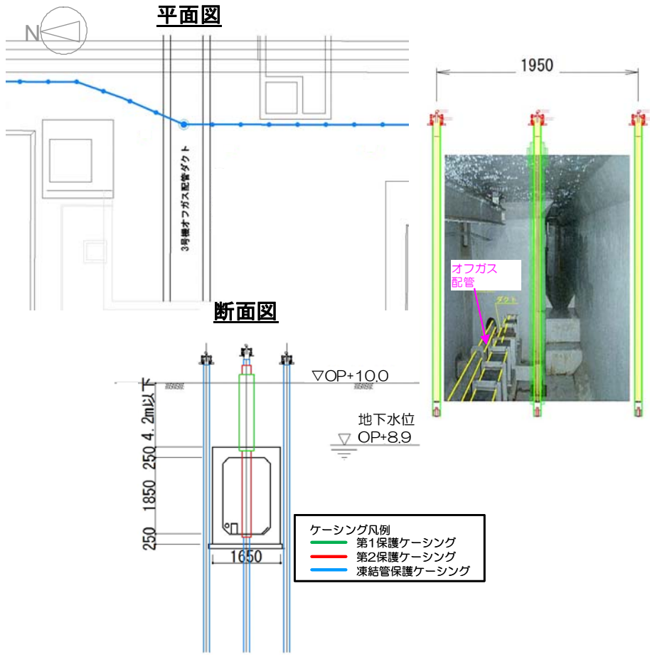
図 1 4 - 1 2 3号機オフガス配管ダクト（北側） 施工方法（貫通施工）
