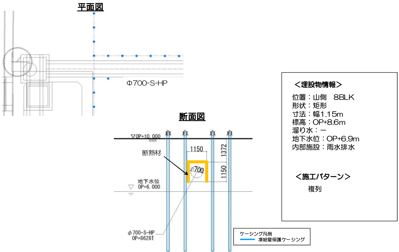
図 1 4 - 2 4 排水ヒューム管② 施工方法（複列施工）
