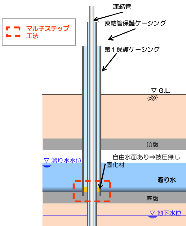
頂版単純貫通・底版マルチステップ工法 (内部充填工を実施しない場合の例)
