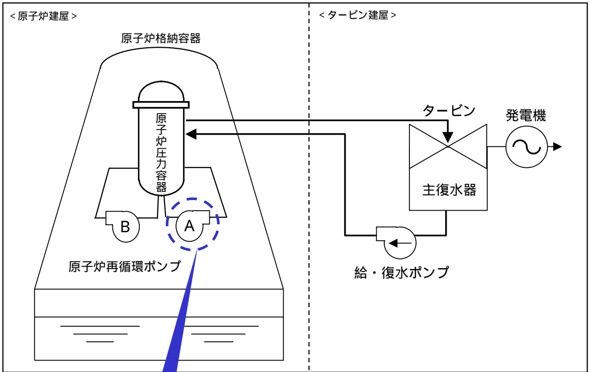
系統概略図
