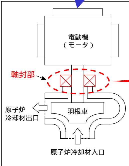
原子炉再循環ポンプ概略図
