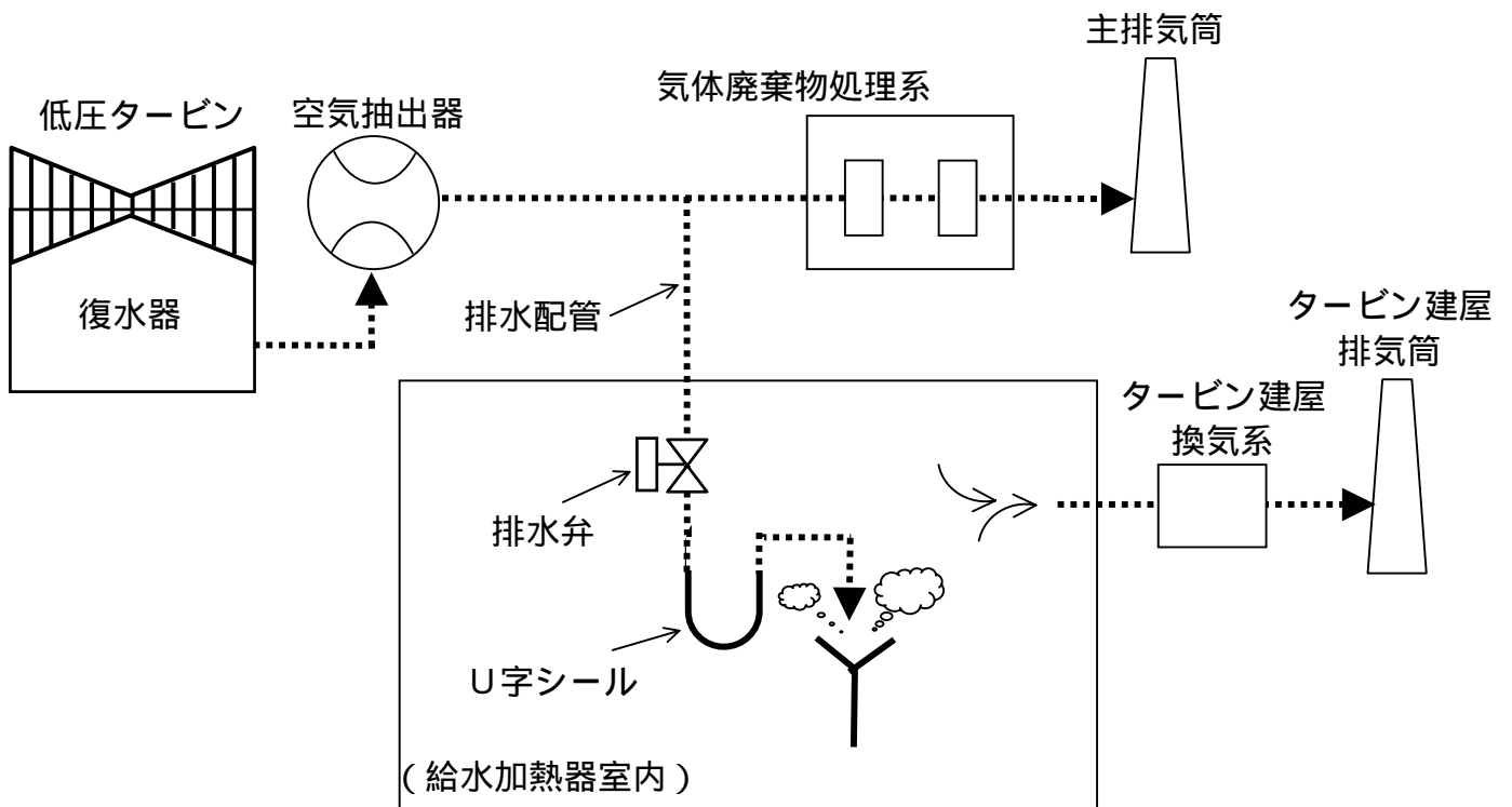
4号機タービン建屋換気系モニタの指示値上昇の概要図
