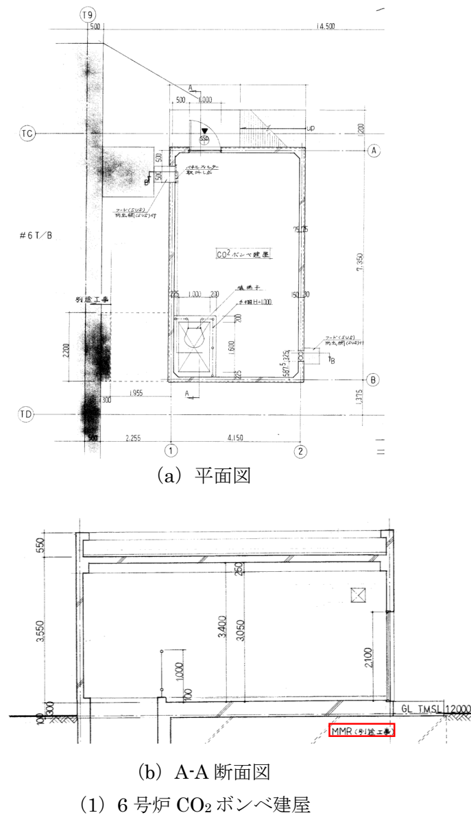
第4図 下位クラス施設の接地状況
