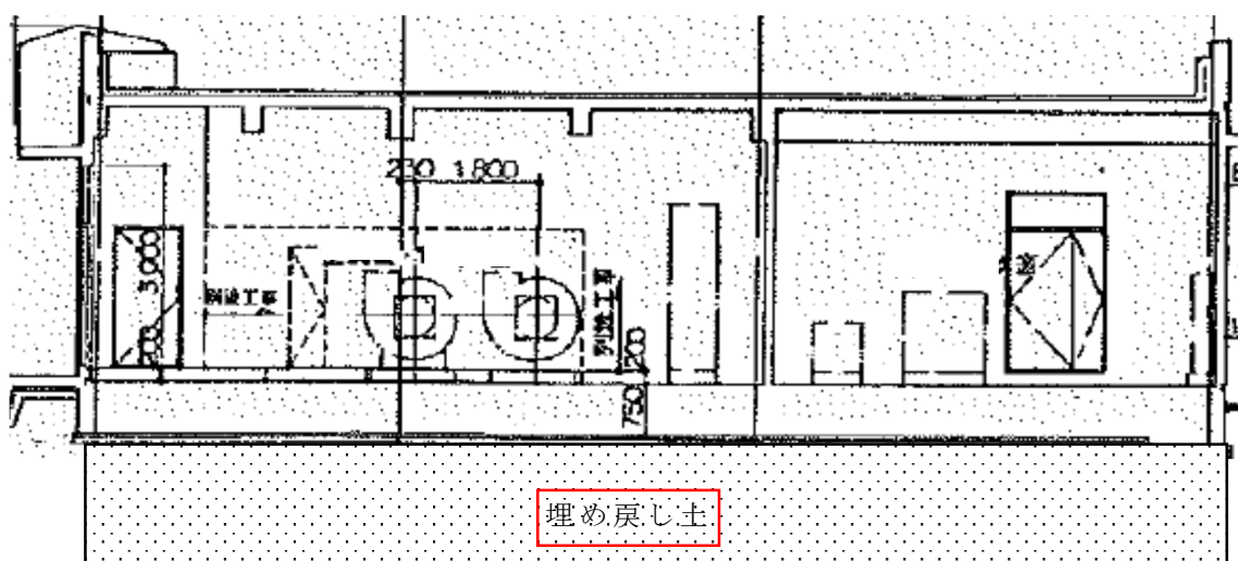
第9図 5号炉主排気モニタ建屋の接地状況
