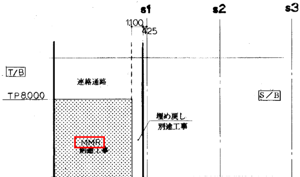
(b) A-A 断面図
