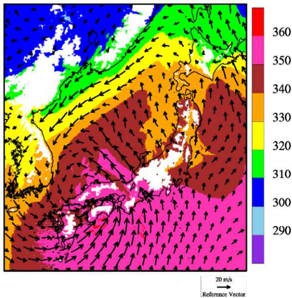
図 11 1999/09/24 F3 事例における気象場と突風関連指数 (左) 500 m 高度における風向・風速および相当温位 (単位: K) (左下) SReH, (右下) 最大 CAPE
