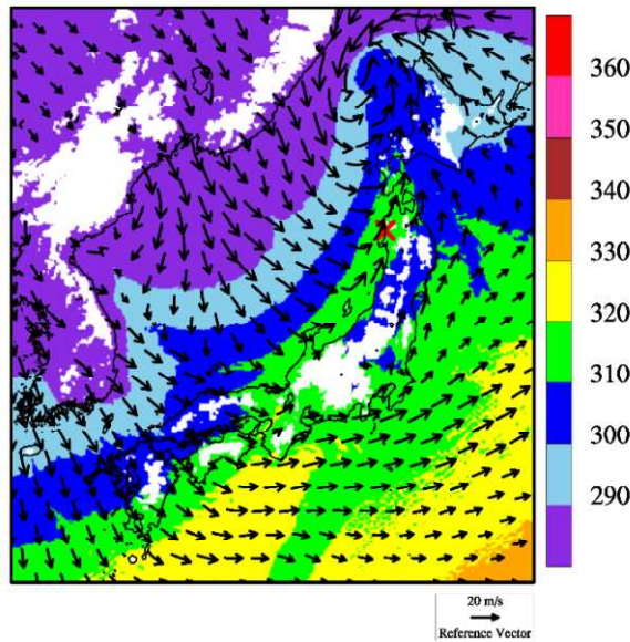
図 18 1999/11/25 F1-F2 事例における気象場と突風関連指数（左）500 m 高度における風向・風速および相当温位（単位：K）（左下）SReH，（右下）最大CAPE
