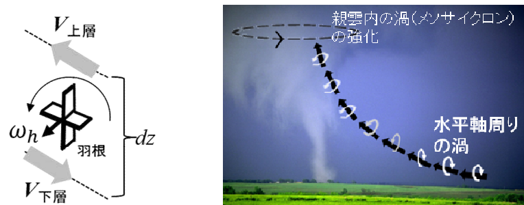
図 6 SReH の算出概念
