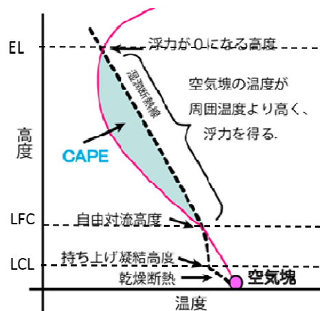
図 7 CAPE の算出概念
