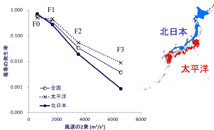
図 24 各 F スケールの発生率
