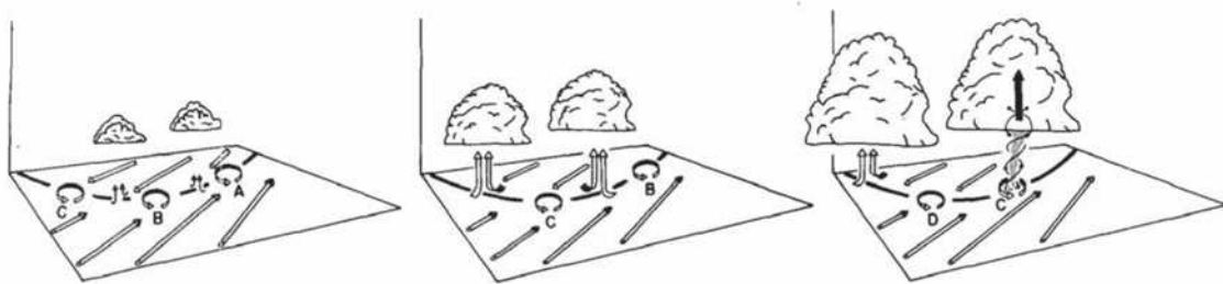
図4 局地前線に伴う竜巻の発生機構に関する模式図 (上向きの黒い⇒が上昇気流を表す)
