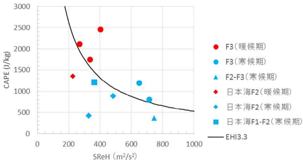
図 19 SReH と最大 CAPE の関係
