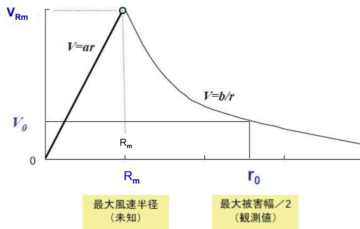
図 1 竜巻半径と風速との関係 (ランキン渦モデルの場合)
