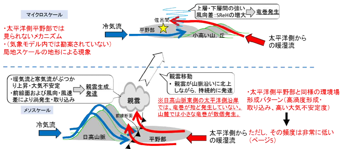
図 29 佐呂間竜巻の発生メカニズムに関する模式図
