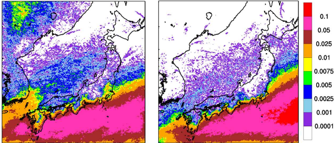
図 21 同時超過頻度分布（単位：%，F3 規模以上を対象；左：暖候期，右：寒候期） （実績ベースの閾値（SReH：250 m 2 /s 2 ，最大 CAPE：1600 J/kg（暖）600 J/kg（寒）））
