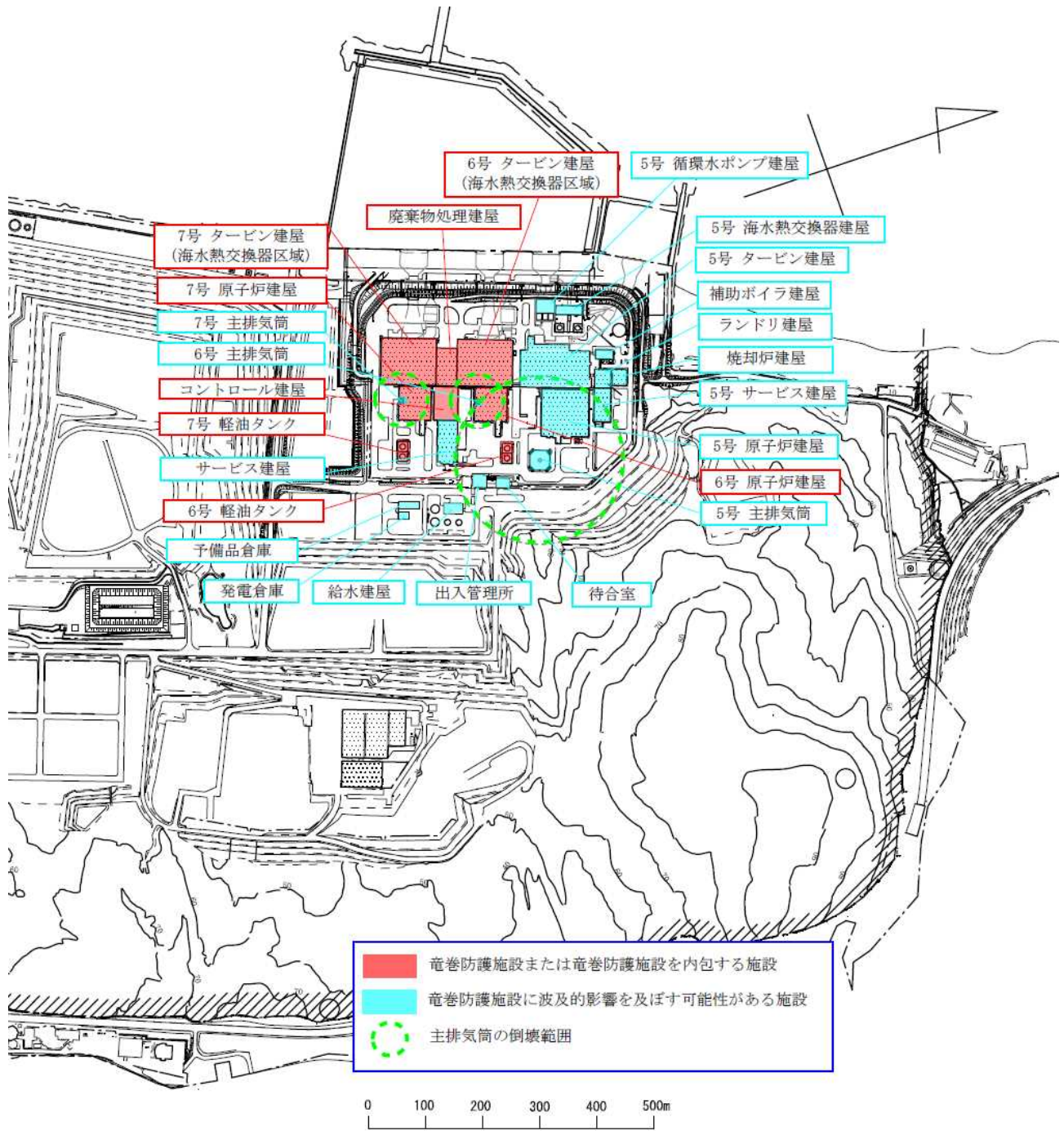
図1.4.3 倒壊により竜巻防護施設が損傷する可能性がある施設の抽出
