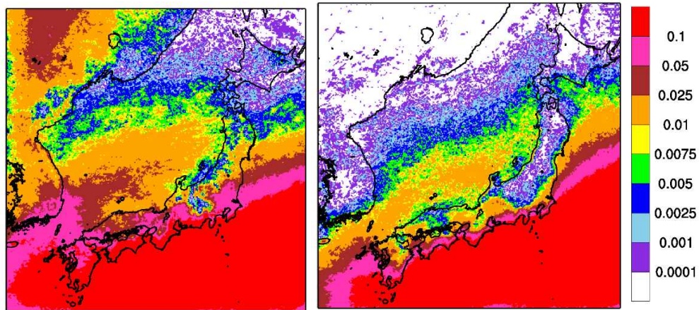
図 25 同時超過頻度分布（単位：%，F2 規模以上を対象；左：暖候期，右：寒候期） (SReH の閾値：200 \text{m}^2/\text{s}^2 ，最大 CAPE の閾値：1000 J/kg（暖）350 J/kg（寒））
