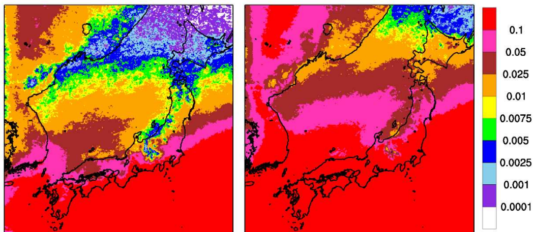
図 28 超過頻度分布（単位は %；通年；EHI の閾値：（左）1.5，（右）0.8）
