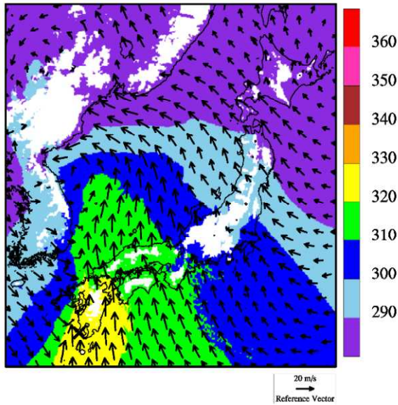
図 14 1990/02/19 F2-F3 事例における気象場と突風関連指数（左）500 m 高度における風向・風速および相当温位（単位：K）（左下）SReH，（右下）最大 CAPE
