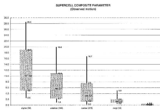
図 B-3 SCP に対する箱ひげ図 (sigtor は F2 規模以上, weaktor は F1 規模以下, nontor は非竜巻, mrg1 はややスーパーセル化したストーム, nonsuper は非スーパーセルストームを表し、括弧内の数字は事例数を表す。箱ひげ図の意味は図 B-2 と同じ。)
