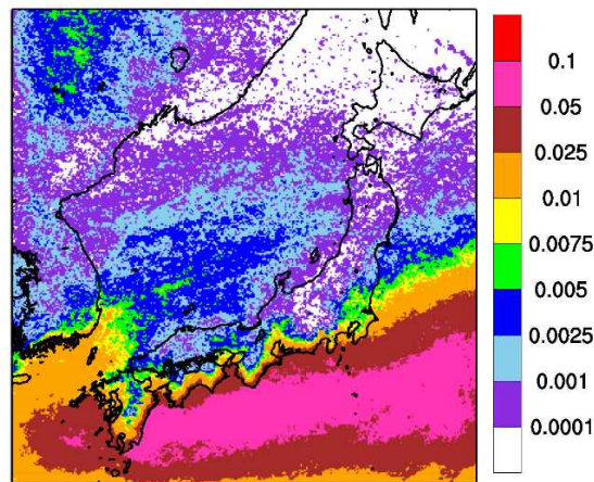
図 23 超過頻度分布 (単位は % ; 通年 ; EHI の閾値 : 3.3)
