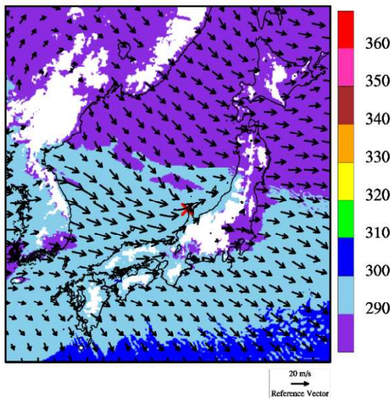
図 16 1990/04/06 F2 事例における気象場と突風関連指数 (左) 500 m 高度における風向・風速および相当温位 (単位: K) (左下) SReH, (右下) 最大 CAPE
