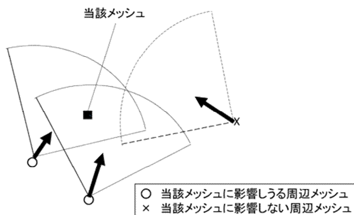
図 8 最大 CAPE 値の抽出方法の概念図
