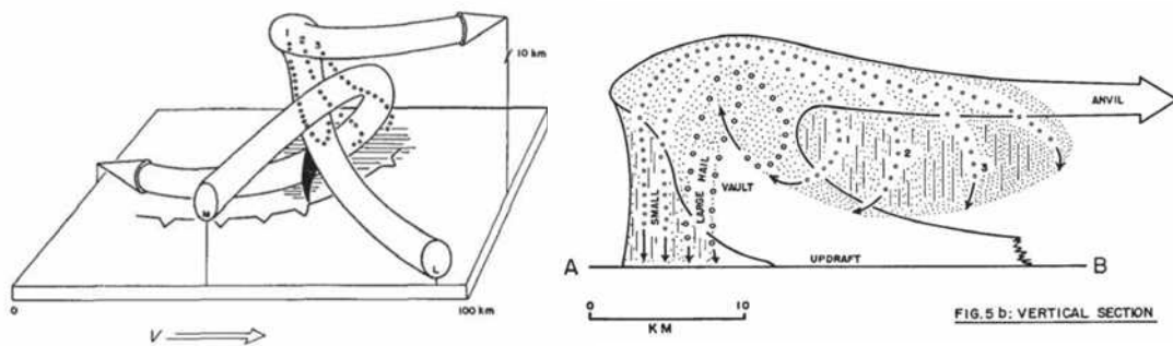
図5 スーパーセル型雷雨の構造 (左: 風況場, 右: 鉛直断面構造) (左図の黒塗り部は竜巻発生箇所を表す。)
