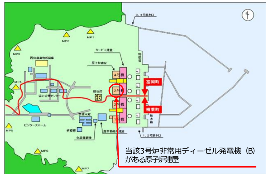
福島第二原子力発電所 現場概略図
